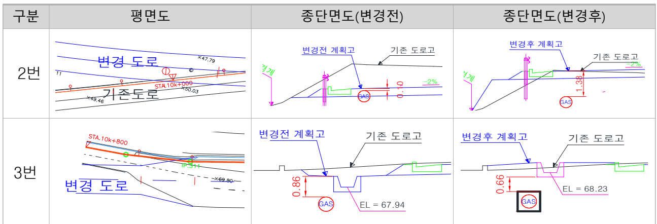
【그림 2. 저축 2, 3번 구간 변경 전·후 종단면도】
